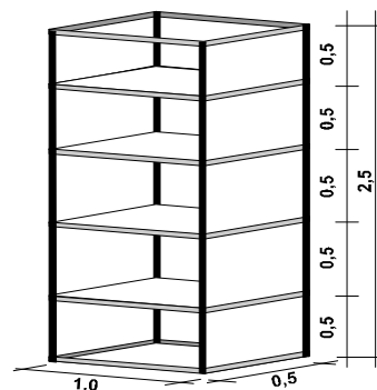
REGAŁ (25)
